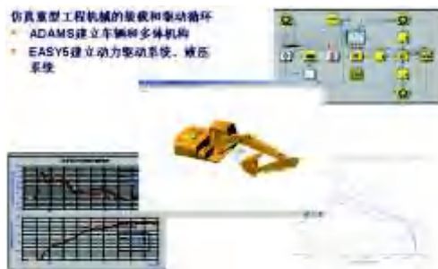
Easy5与Adams集成仿真重型工程机械模型
